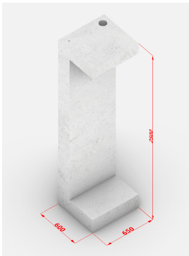
Πίλλαρ ΔΕΗ - Μονό Ρολόι Ανοιχτού Τύπου 65x60x250cm
