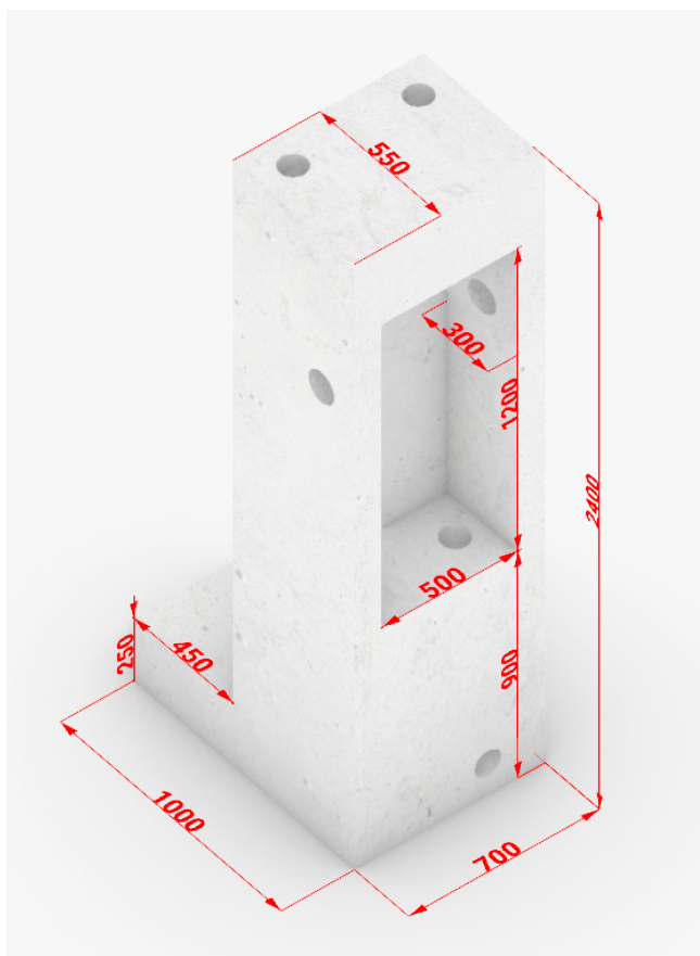
Πίλλαρ ΔΕΗ - Μονό Ρολόι Κλειστού Τύπου 70x100x240cm
